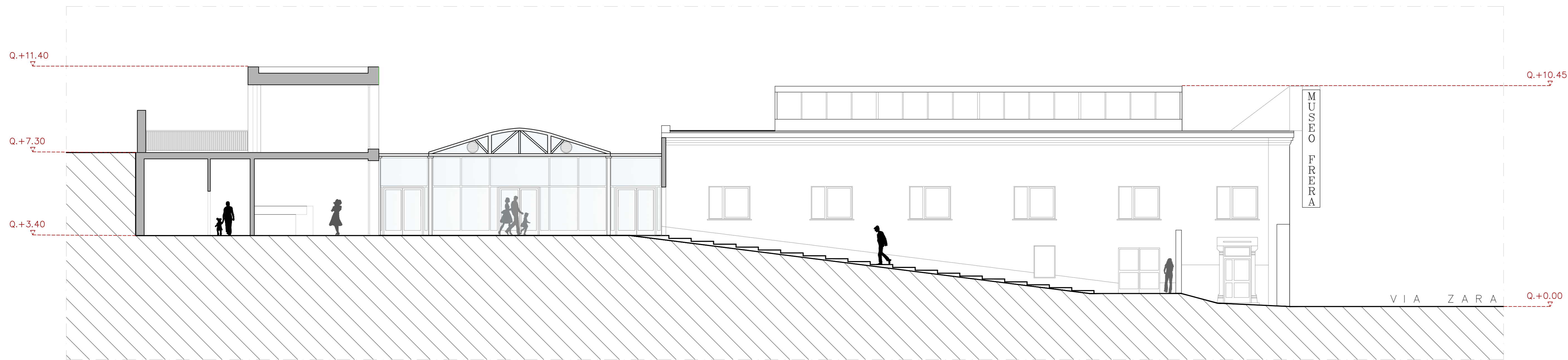
PROSPETTO NORD-OVEST - SEZIONE FF'
